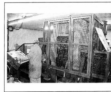
Unité de production de Baume-les-Dames : forgeage à froid de pinces, 2.000 pièces par jour
